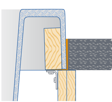
SILGRANIT®: modul uprostred
