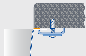
Nerez: zabudovanie drezov pod pracovnú dosku
