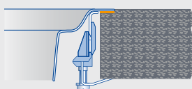
Nerez: zabudovanie do roviny s pracovnou doskou
