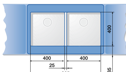
BLANCO ANDANO 400/400-U
