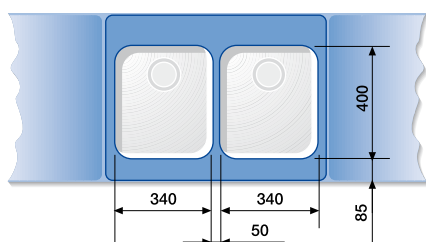
BLANCO SUPRA 340-U + BLANCO SUPRA 340-U
