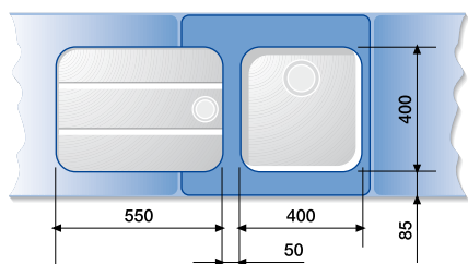
BLANCO SUPRA 550-T + BLANCO SUPRA 400-U
