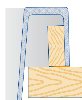
SILGRANIT®: modul naložený
