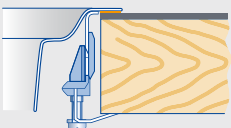
Nerez: zabudovanie zhora alebo plocho naložený
