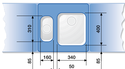
BLANCO SUPRA 160-U + BLANCO SUPRA 340-U
