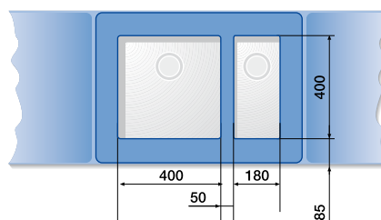
BLANCO ANDANO 400-U + BLANCO ANDANO 180-U
