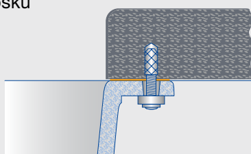
SILGRANIT®: Vaničky pod pracovnú dosku
