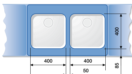
BLANCO SUPRA 400-U + BLANCO SUPRA 400-U
