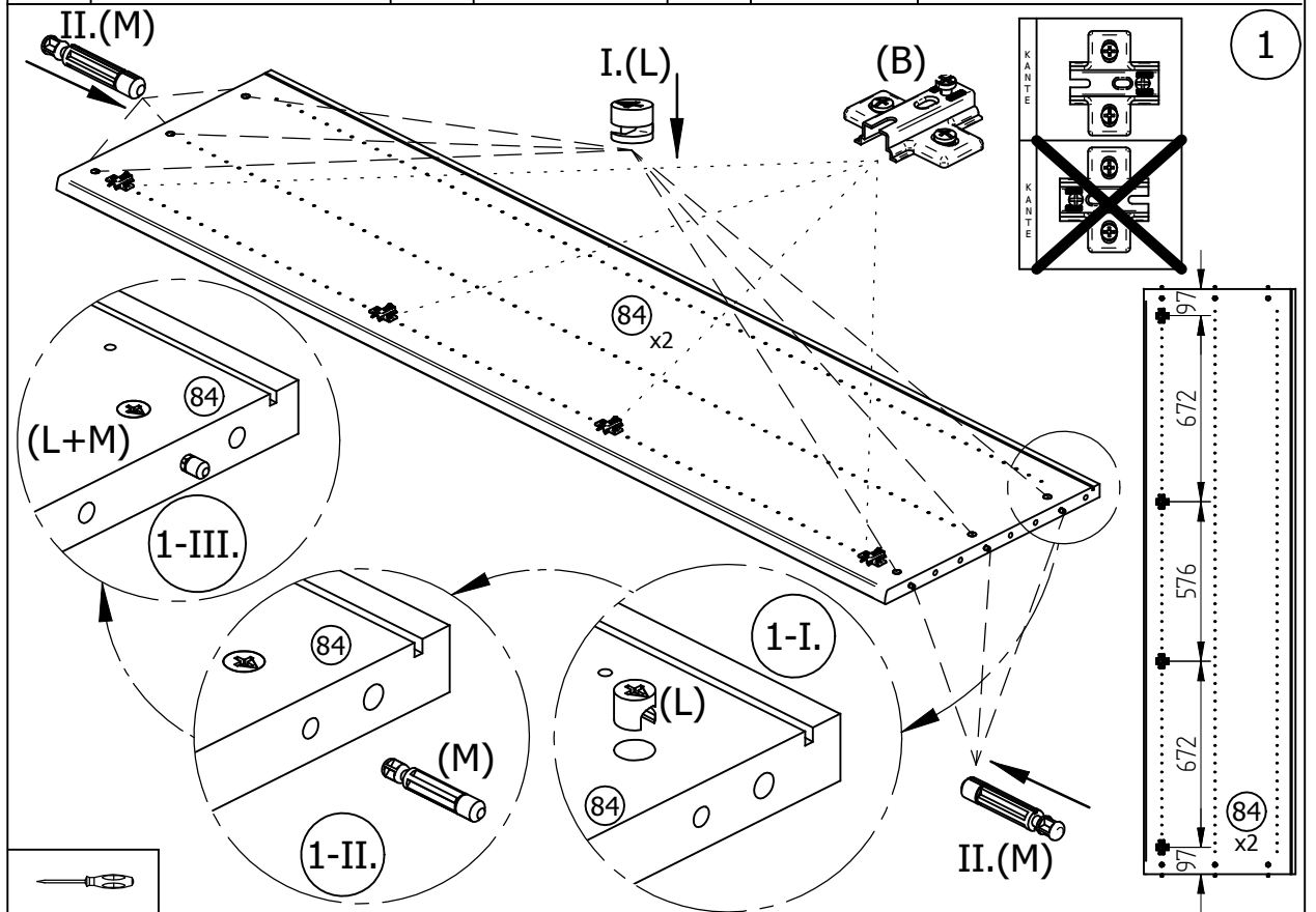
MONTAGESCHABLONE
